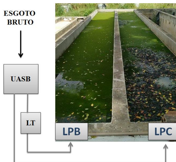
Figura I- Esquema do sistema experimental formado por um reator UASB, tratando esgoto bruto, seguido de lagoa com alimentação em fluxo contínuo (LPC) e lagoa com alimentação em batelada (LPB), através de lagoa de transbordo (LT).
